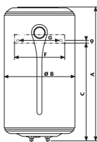
Вид спереди
